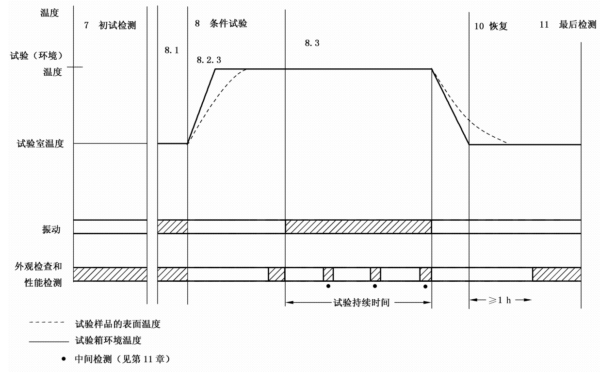
图 1 非散热试验样品试验曲线图
